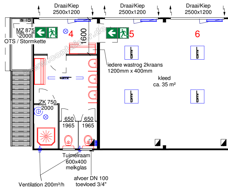
Bouvenverdieping M: 1 : 100
