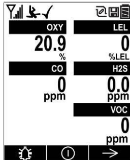
Vijf sensoren, waaronder PID, met lamptype, correctiefactor en meetgas.
